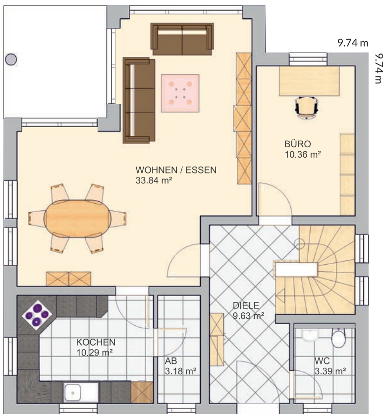
Erdgeschoss
