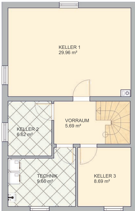
Kellergeschoss
