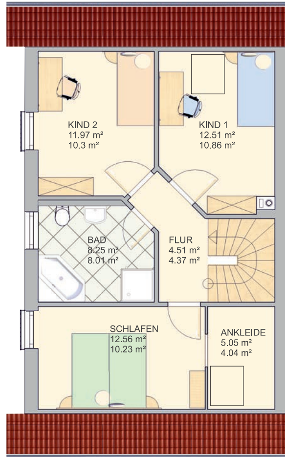
Dachgeschoss
